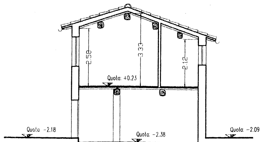
SEZIONE C-C'
