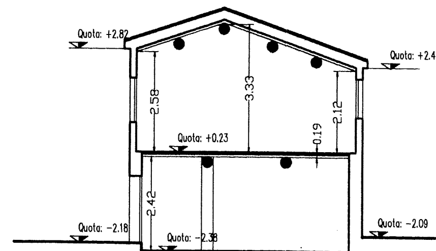
SEZIONE C-C'
