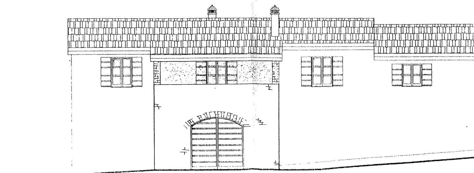
PROSPETTO N-O
