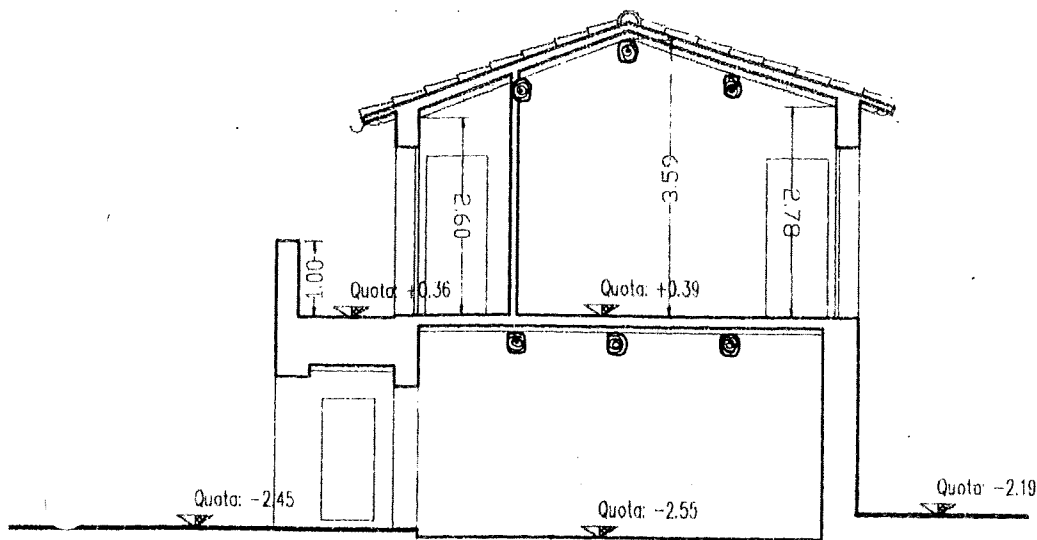
SEZIONE B-B'
