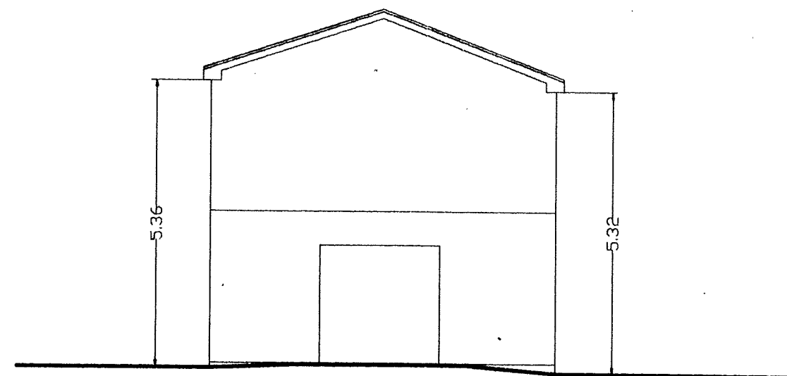
PROSPETTO N-E
